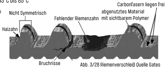
Abb. 3/28 Riemenverschleiß Quelle Gates
