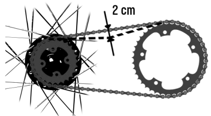
Abb. 4/21 Kettenspannung
