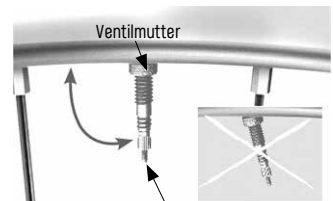
Korrekte Ventilstellung
