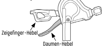
Abb. 3/23 Schalthebeleinheit Umwerfer Quelle Shimano
