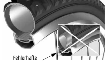
Fehlerhafte Schlauchmontage
